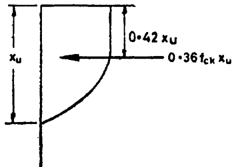
FIG. 4 STRESS BLOCK PARAMETERS
