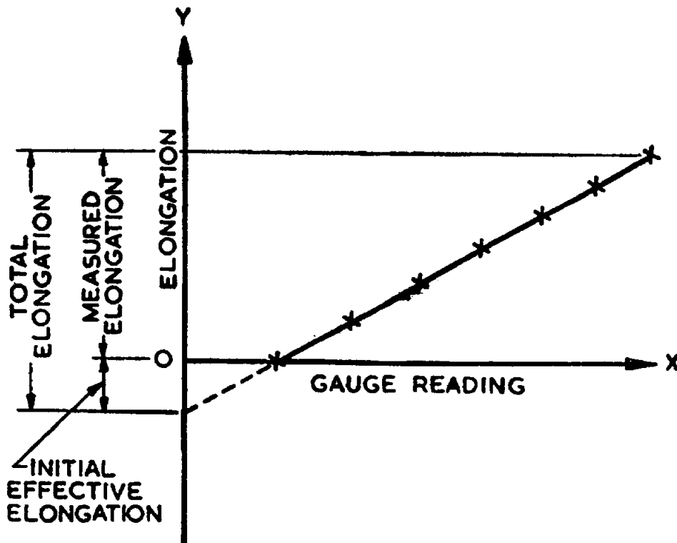
FIG. 2 DETERMINATION OF ACTUAL ELONGATION
